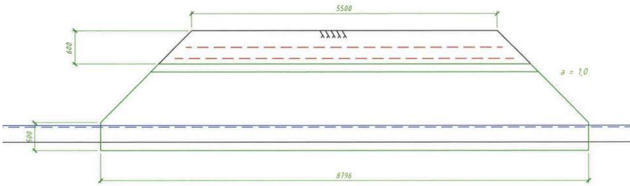
Længdesnit, 1:50 Stålrørsbro, SC-2B
