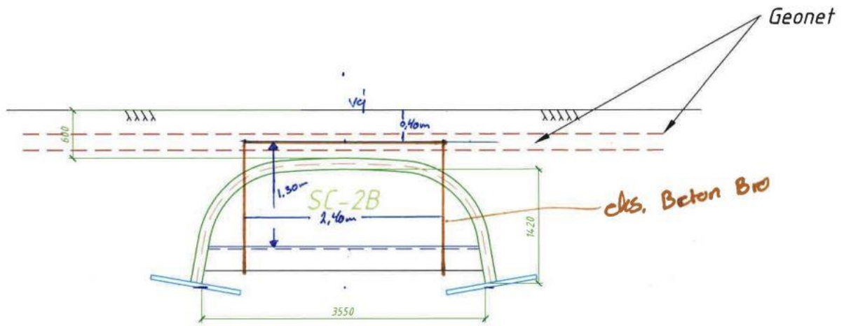
Tværsnit, 1:50 Stålrørsbro, SC-2B
