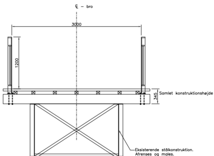
Figur 5. Tværsnit bro.
